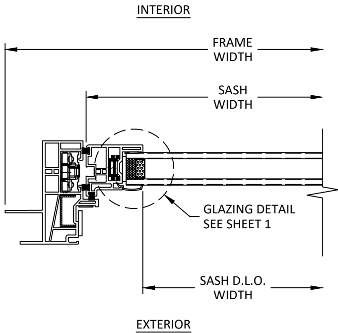
F 4 HORIZONTAL SECTION SASH JAMB
