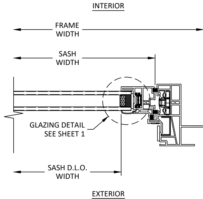
G 4 HORIZONTAL SECTION SASH JAMB
